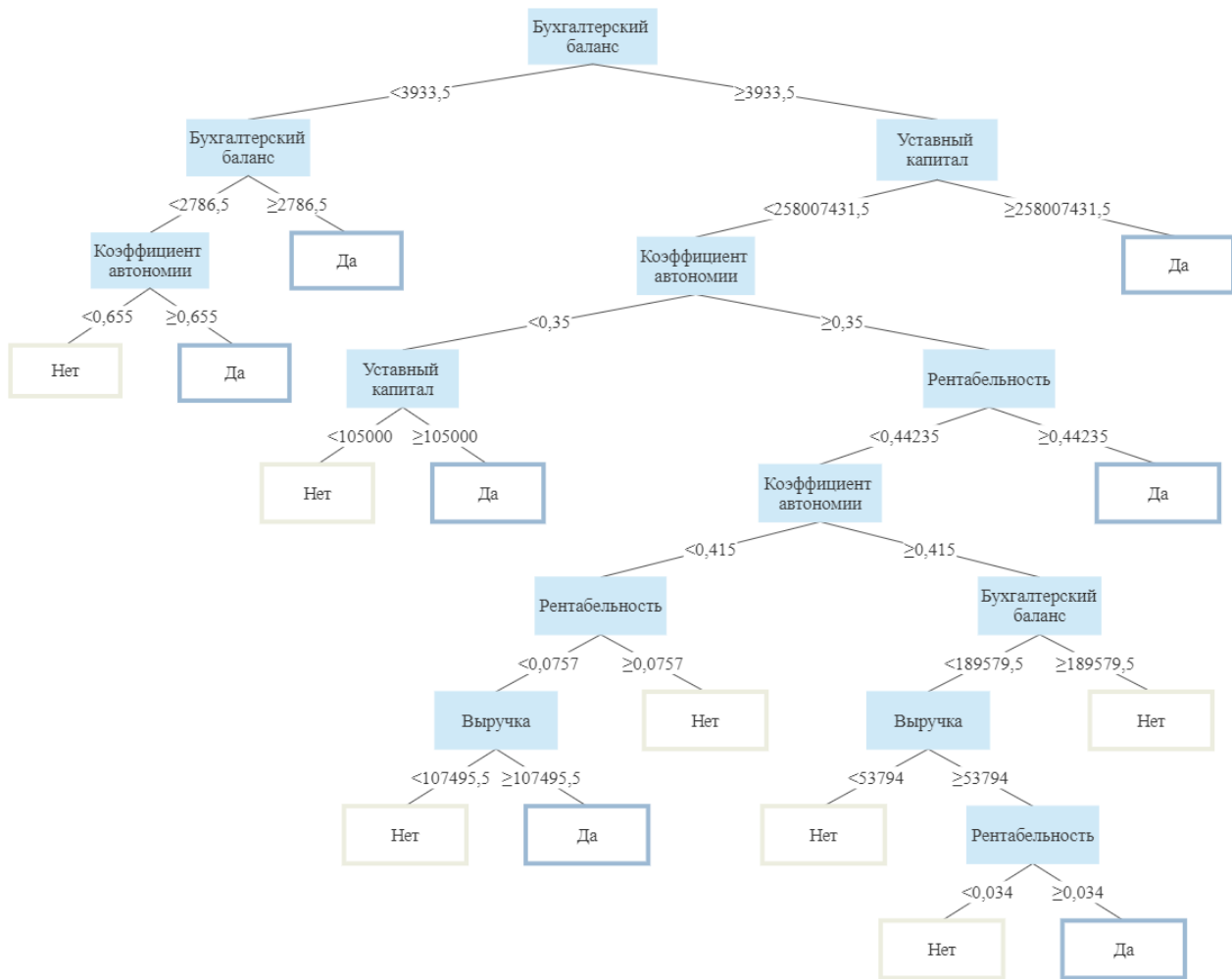
Рисунок 5 – Модель дерева решений по выявлению потенциальных участников нарушений (потенциальный нарушитель / не нарушитель)
