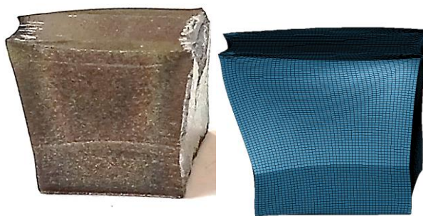
Рисунок 7 – Фотография и результат численной симуляции при скомпенсированном нагружении образца 4 (покрытие располагается справа)
