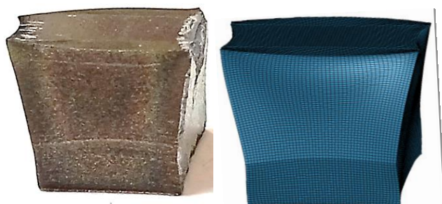
Рисунок 6 – Фотография и результат численной симуляции при одноосном сжатии образца 4 (покрытие располагается справа)
