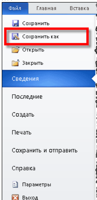
Рисунок 4 - Сохранение файла
