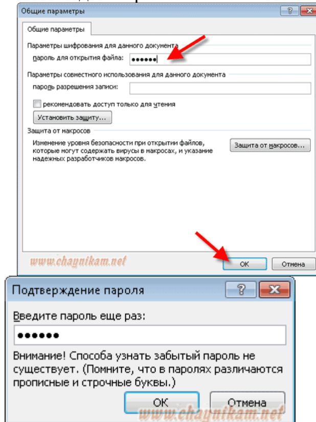
Рисунок 7 - Задание пароля
