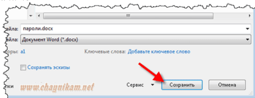
Рисунок 8 - Сохранение файла
